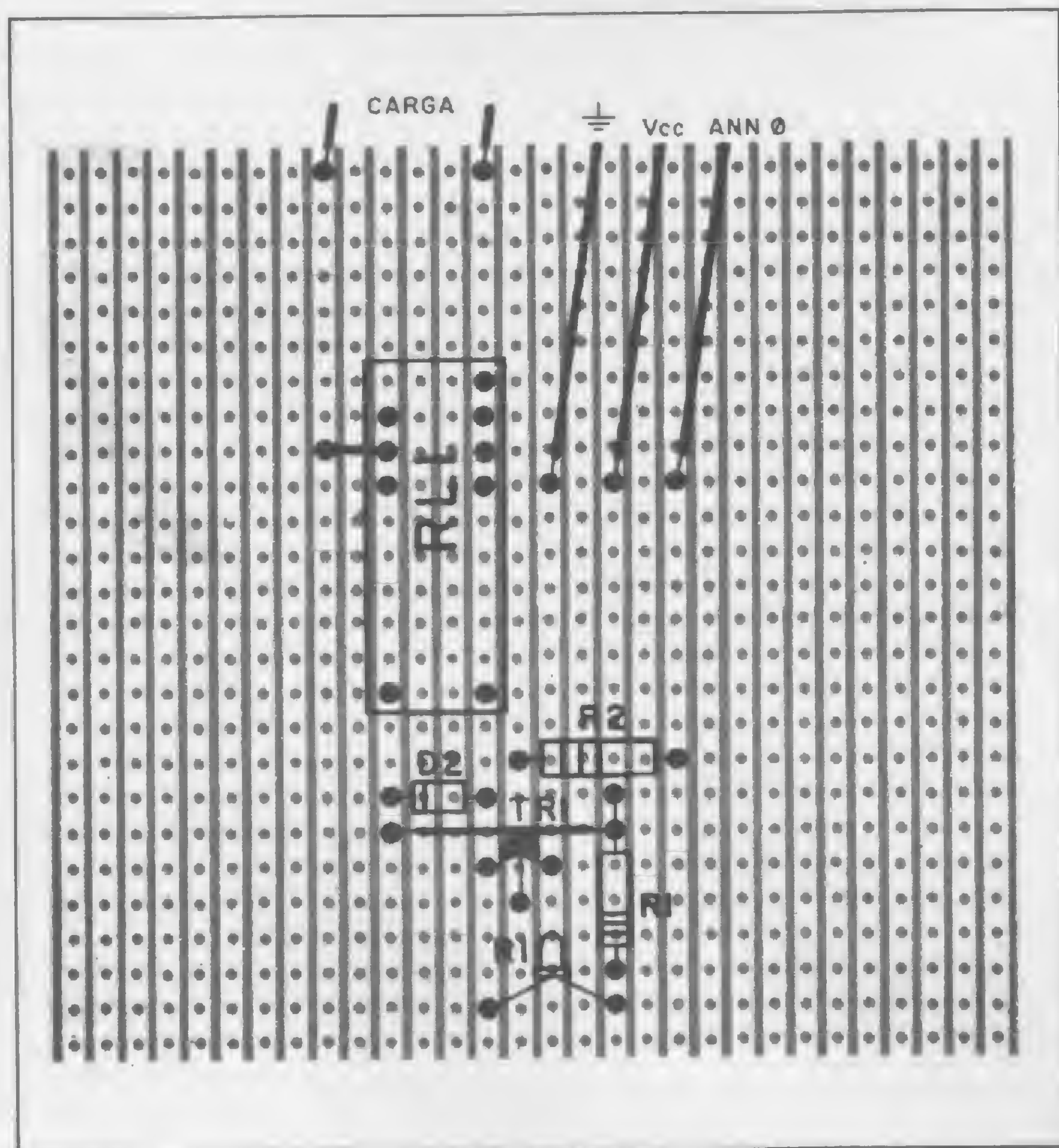
Figura 3 – Placa de circuito impresso universal 12,5 x 7,5, vista pela face dos componentes.
